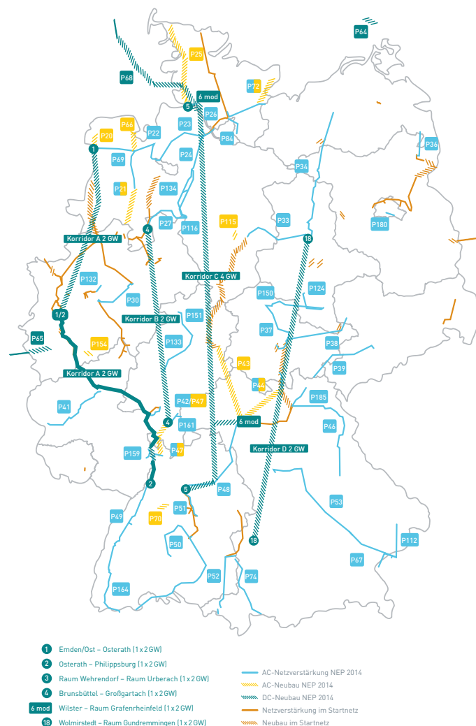
Abb.: geplante HGÜ- Übertragungsnetze Deutschland
