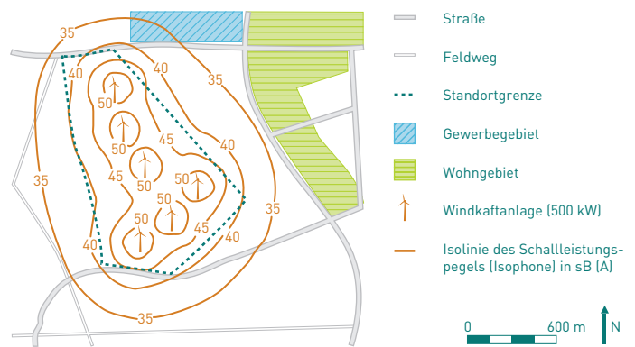
Abb.: Schallpegelausbreitung für einen Windenergiepark
