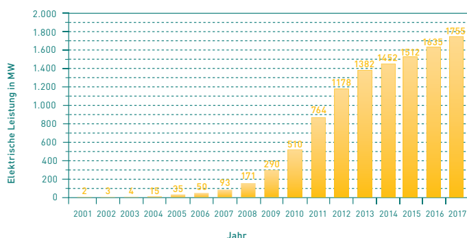
Abb.: Elektrische Leistung Photovoltaik in Sachsen
